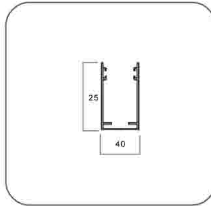
Guías
